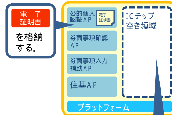
ICチップ内のAP構成
